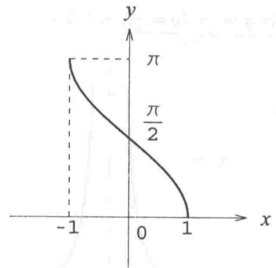
F8*: y = \arccos x
